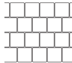
8" Tile Tile Size 195 x 195
